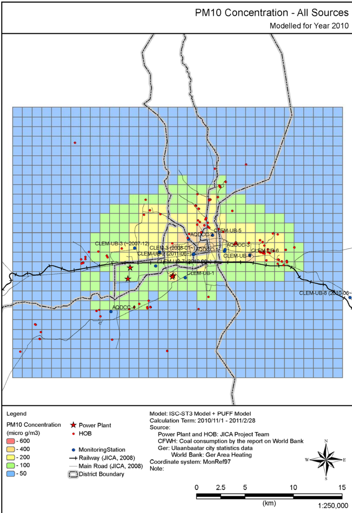
Зураг 2-7. PM 10 -н тархалтын загварчлалын дүн
