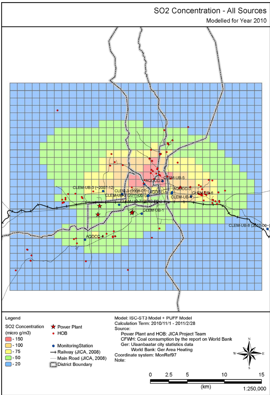
Зураг 2-6. SO 2 -ын тархалтын загварчлалын дүн
